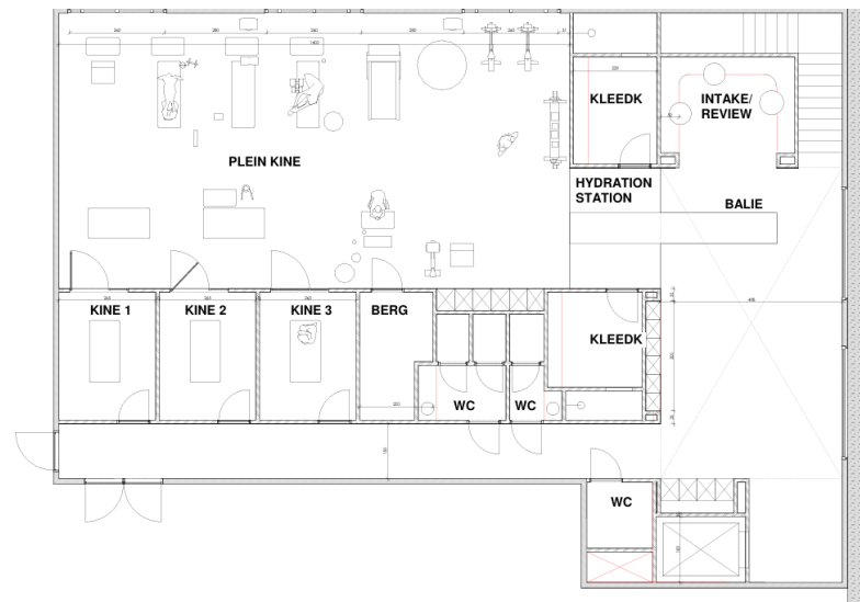
Grondplan gelijkvloers
